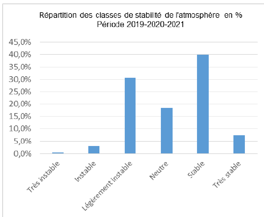
Figure 5 : Répartition des classes de stabilité de Pasquill à Genève-Cointrin (période 2019-2020-2021)
