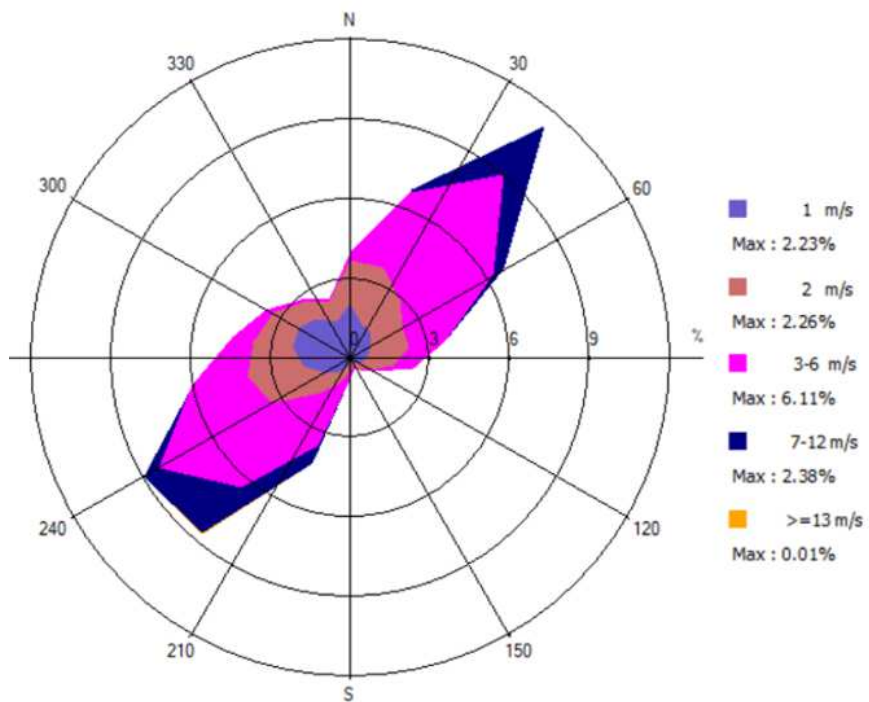
Rose des vents 2020
