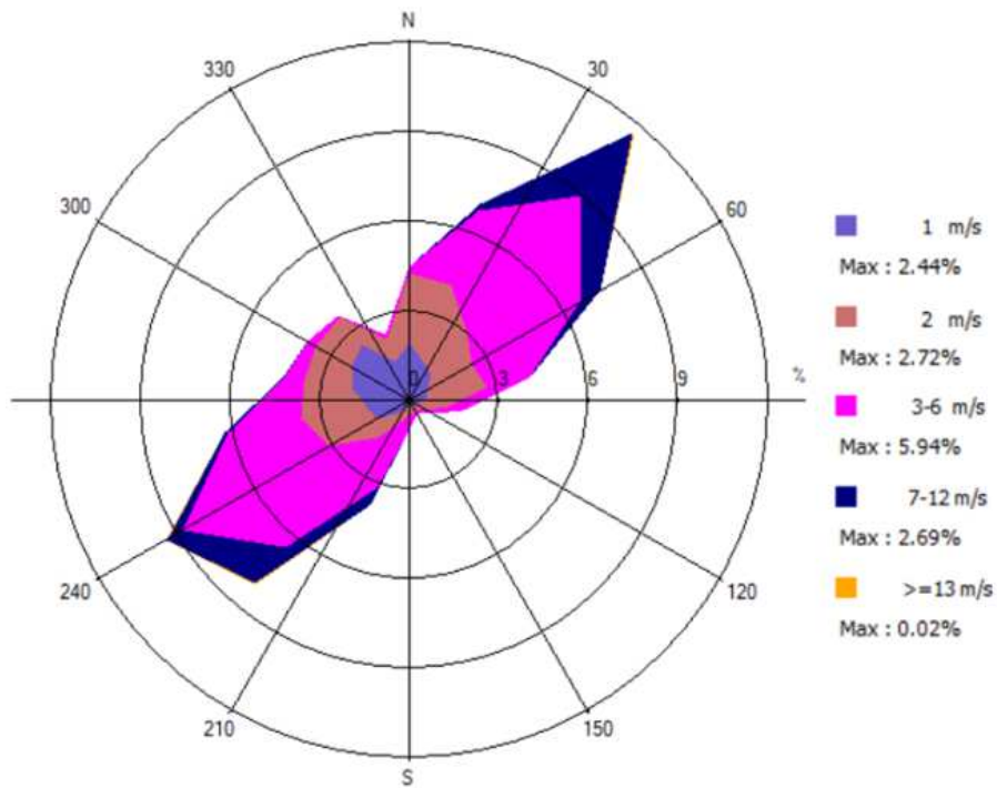
Rose des vents 2019
