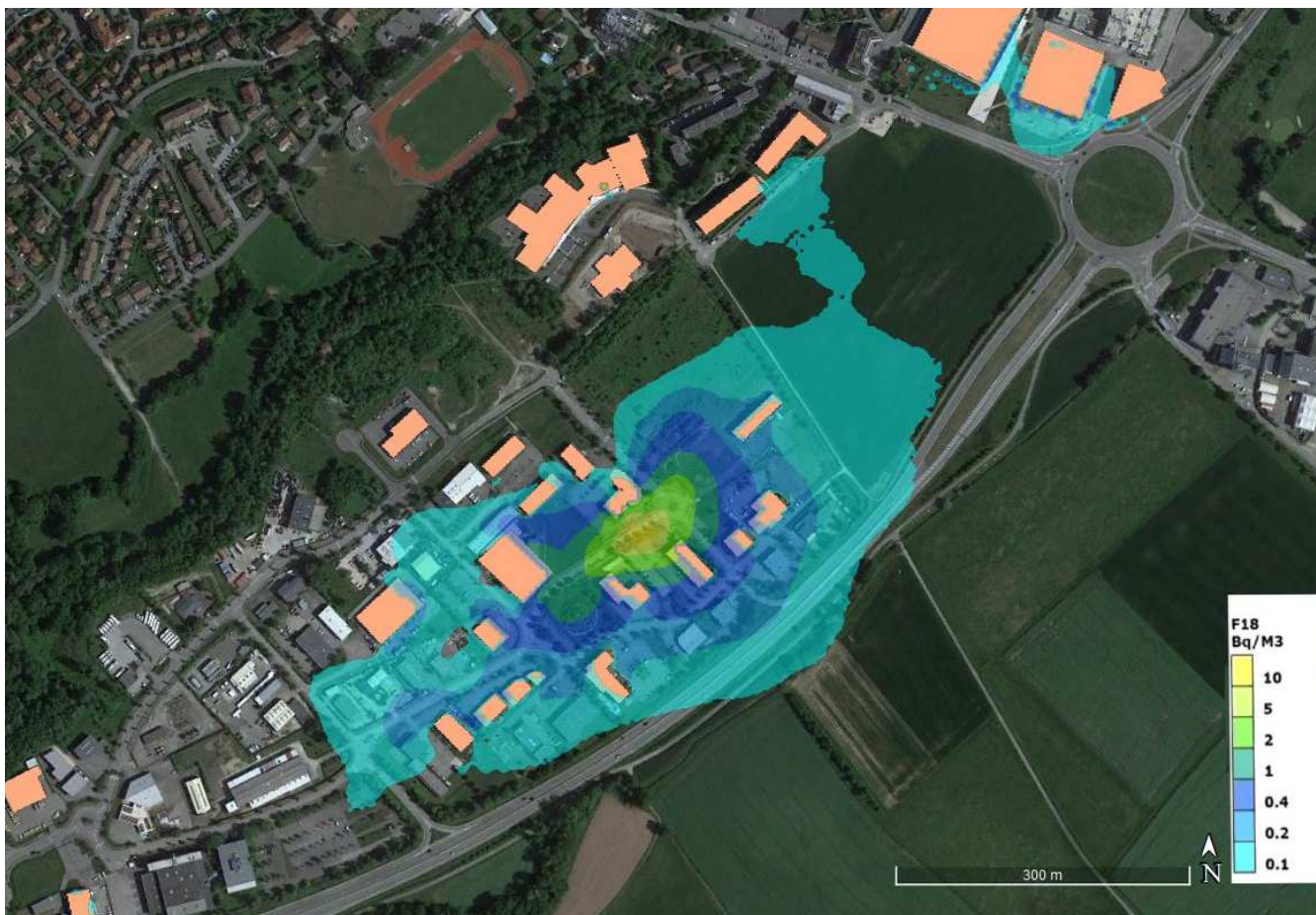
Figure 7 : Concentration moyenne annuelle (Fluor 18 attribuable à A.A.A)
