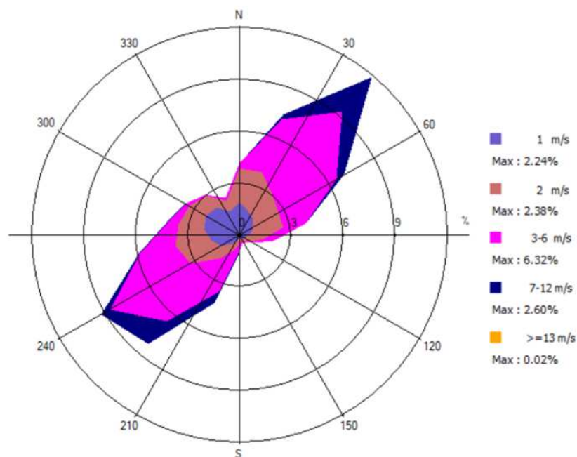
Rose des vents sur la période 2019-2020-2021
