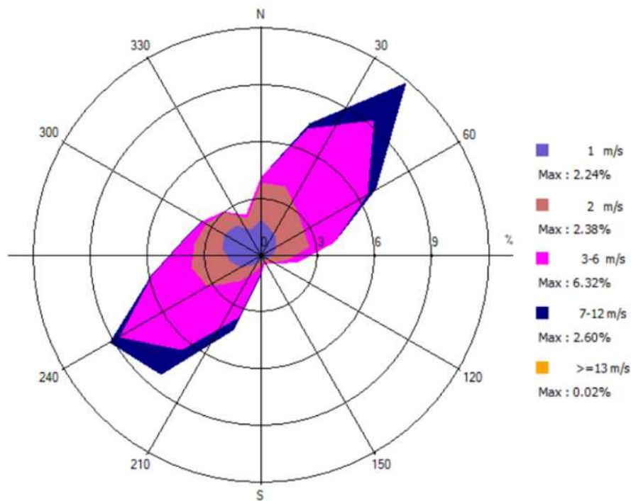
Figure 4 : Rose des vents de Genève-Cointrin (période 2019-2020-2021)
