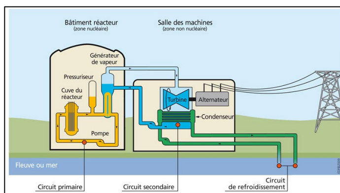
Figure 1: Principe de fonctionnement d'une centrale nucléaire sans tour aéroréfrigérante (circuit dit « ouvert ») (source : IRSN)
